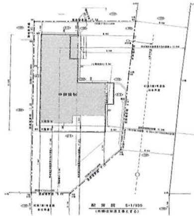
配置図
