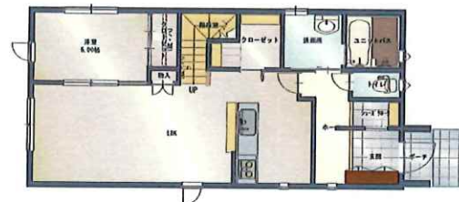
1階
