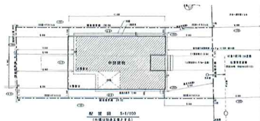
配置図
