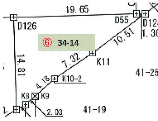
寸法図
