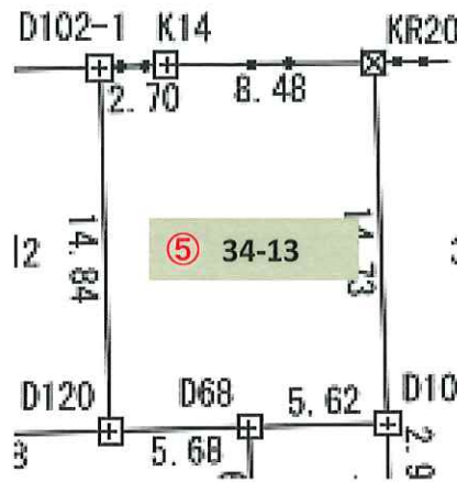
寸法図
