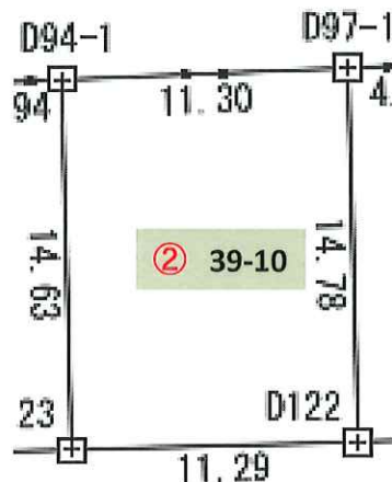
寸法図
