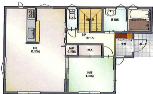
1階
