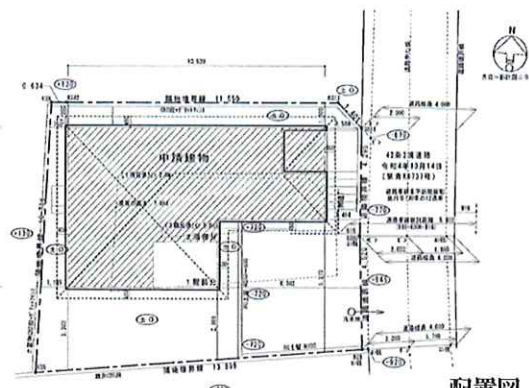
配置図
